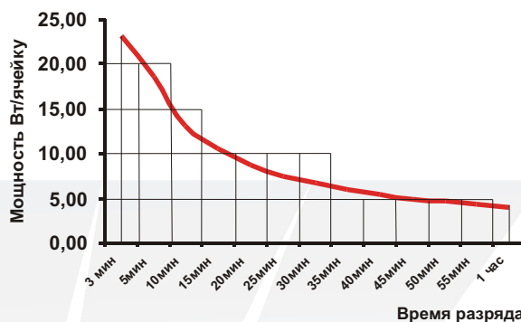
Разряд постоянной мощностью ( U_{кон}=1,7 В T=20 С )
