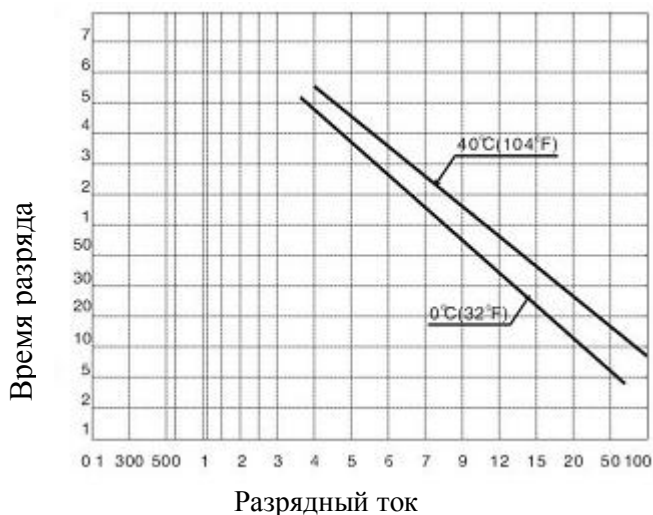
Разрядные характеристики
